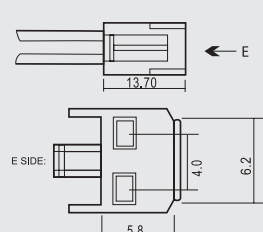
JST-Stecker
